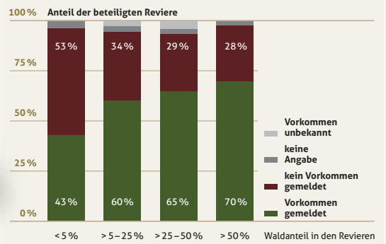
Vorkommen der Waldschnepe in Abhängigkeit vom Waldanteil
